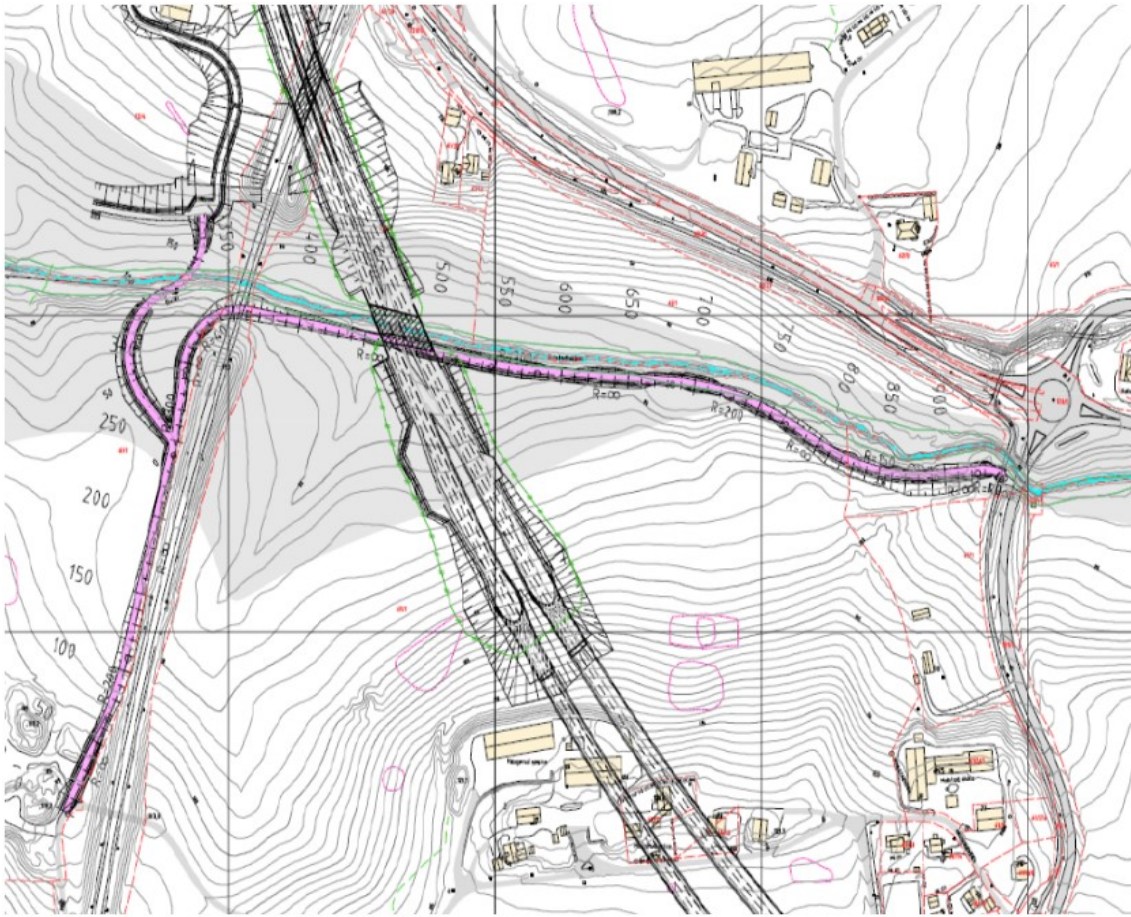
Figur 1. Alternativ 2b i Statens vegvesens mulighetsstudie. Øst for jernbanen går traseen langs Bølstadbekkens sørside. Ny trasé for E18 krysser sykkelveien på jorden ved Haugerud. Plassering av tunnelåpningen for ny E18 er vist i midten av kartet.
